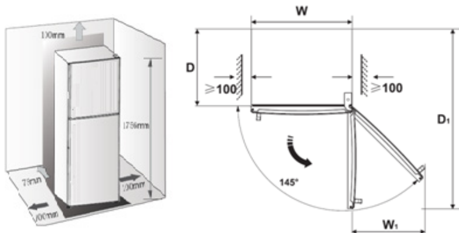
Рисунок-схема рекомендуемого размещения холодильника DR 180
