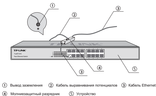
Рисунок 3-4 Выравнивание потенциалов
