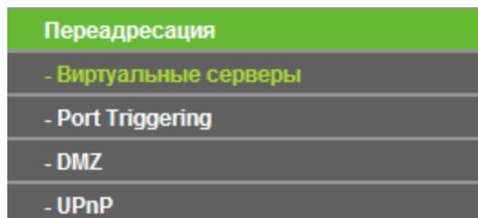
Рис. 4-45 Меню Переадресация
