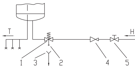
Montāžas shēma
